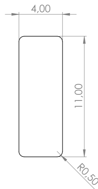
Carta de Pontuação Vista Frontal Esc: 1/2
