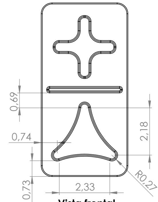
Vista frontal Peça 3
