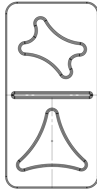
Vista frontal Peça 7
