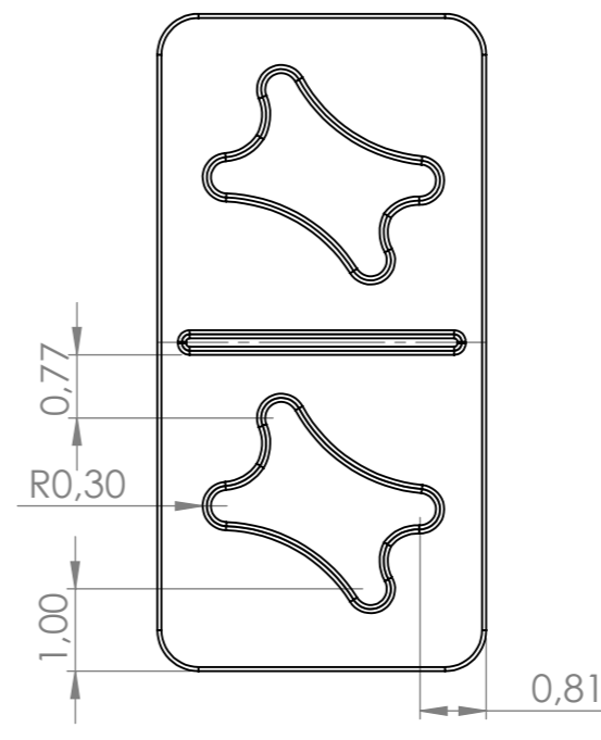
Vista frontal Peça 5
