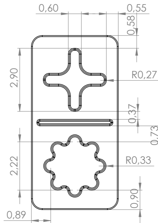
Vista frontal Peça 2
