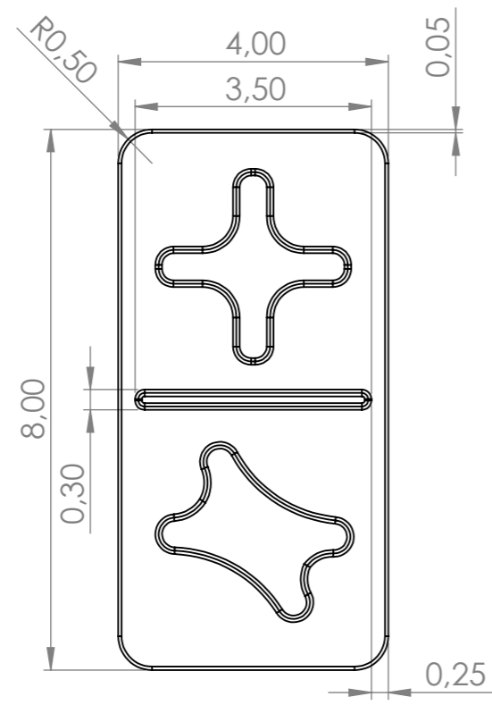
Vista frontal Peça 1
