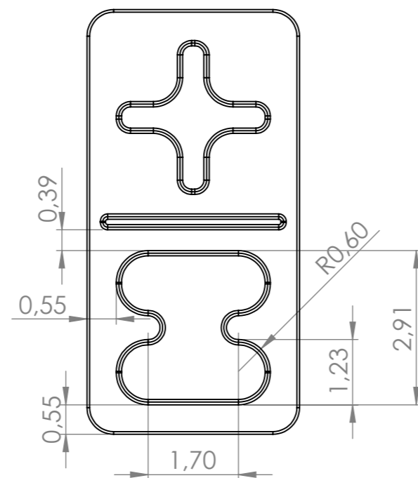
Vista frontal Peça 4
